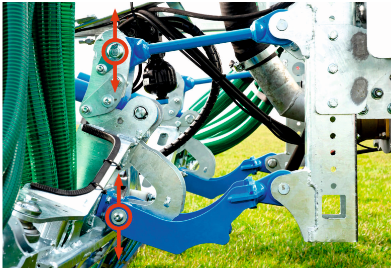
Asennus Bomechin pikavaihtojärjestelmällä
